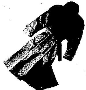
PARA MUJER
