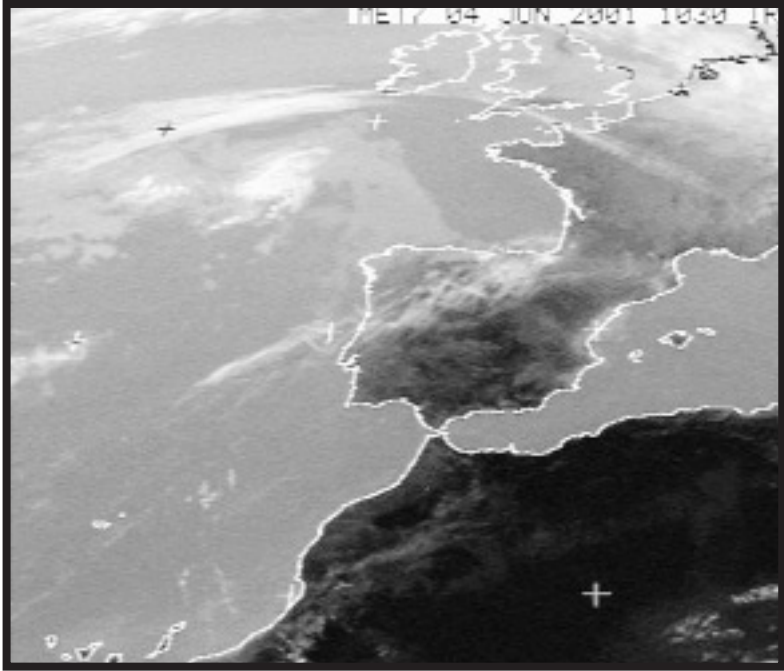
Imagen tomada por el satélite Meteosat ayer por la mañana.
